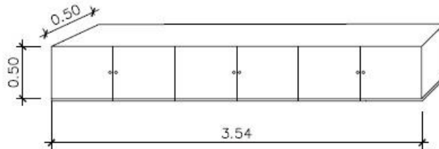
Vista frontal armário aéreo – Sala de som
