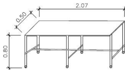
Vista frontal Mesa (a) Móvel – Estúdio de Som
