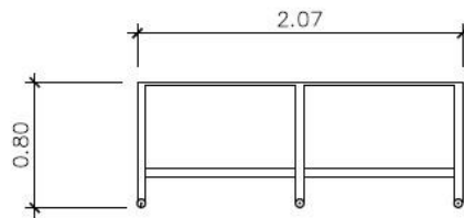
Planta baixa Mesa (a) Móvel – Estúdio de Som
